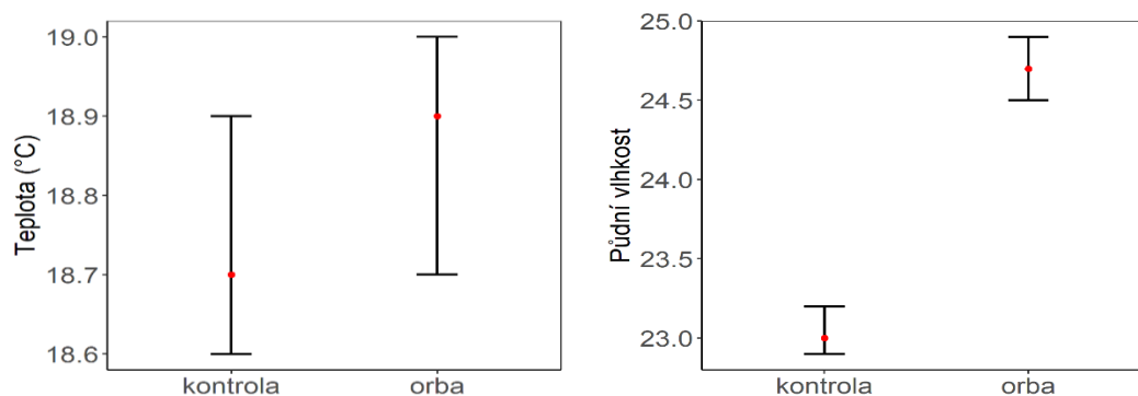
Obr. 84–85: Srovnání průměrné půdní vlhkosti mezi plochami, kde probíhala každoroční orba a kontrolními plochami bez zásahu. Chybové úsečky znázorňují 95 % konfidenční intervaly.
