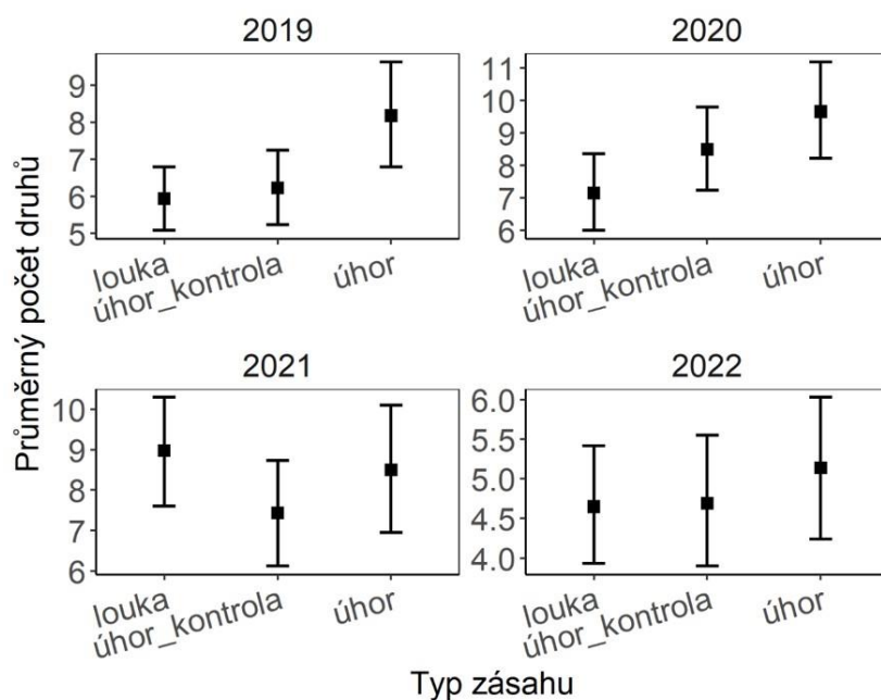
Obr. 69. Změna průměrného počtu druhů brouků v průběhu čtyř let v jednotlivých experimentálních plochách (úhor: aplikace orby jednou za tři roky, úhor-kontrola: neoraná luční plocha přímo navazující na úhor, louka: vzdálená neoraná luční plocha). Čtverec uprostřed naznačuje průměr. Chybové úsečky ukazují 95 % konfidenční interval.
