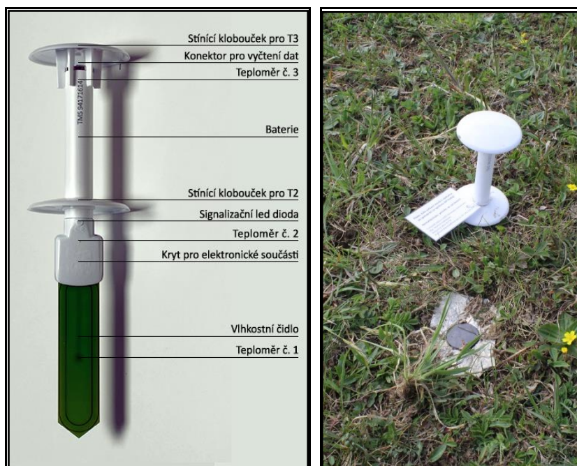
Obr. 27, 28: Nová generace základní verze TMS dataloggeru pro měření teploty vzduchu a půdy a vlhkosti půdy (vlevo schéma s popisem, vpravo čidlo umístěné na lokalitě s informačním štítkem).
