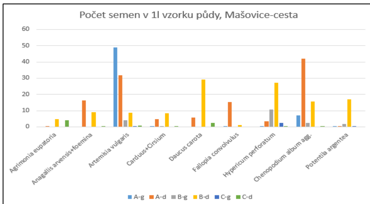
Obr. 56: Srovnání převažujících druhů v semenné bance pro lokalitu Mašovice – u cesty. A, B, C = varianty pokusu; g = vyrostlé semenáčky, d = dormantní semena dohledaná nevyklíčená. Graf zobrazuje pouze 9 taxonů s nejvyšším celkovým počtem nalezených semen a semenáčků (alespoň 10 kusů).
