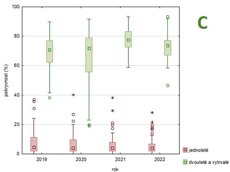
Obr. 53, 54 a 55: Struktura vegetace dle zastoupení jednoletých a vytrvalých druhů rostlin.
