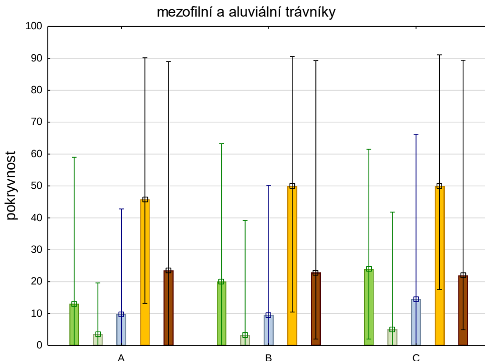
Obr. 27, 28 a 29: Pokryvnosti vybraných funkčních skupin rostlin dle jejich významu v zemědělství (legenda je na předchozí straně), každý sloupec ukazuje průměr (výška sloupce) a úsečky pro minimální a maximální pokryvnost.
