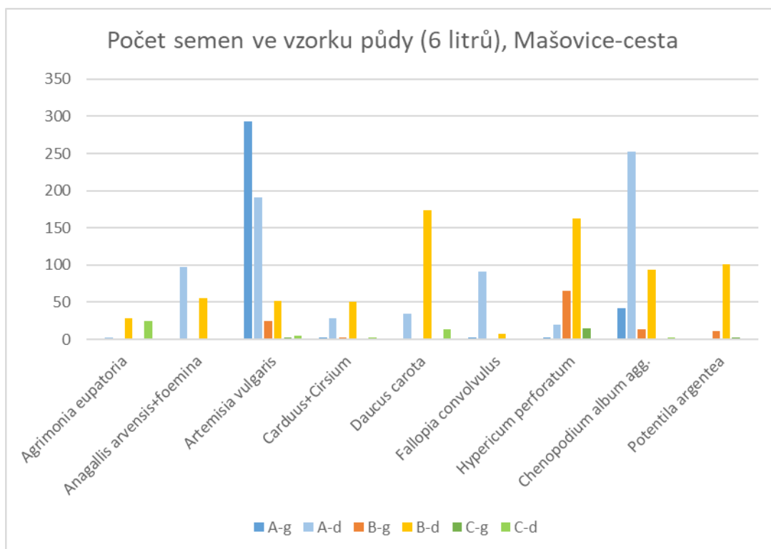
Obr. 37: Počty nalezených semen ve vzorku půdy na lokalitě Mašovice – u cesty. Zobrazeno pouze 9 taxonů s nejvyšším celkovým počtem nalezených semen nebo semenáček (alespoň 50 kusů). A, B, C = varianty pokusu; g = vyrostlé semenáčky, d = dormantní semena.
