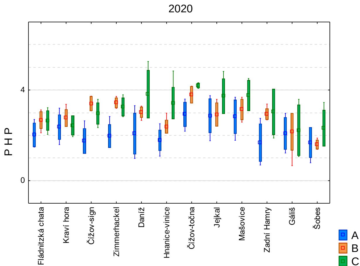
Obr. 36: Vypočítané hodnoty PHP pro jednotlivé lokality v roce 2020.
