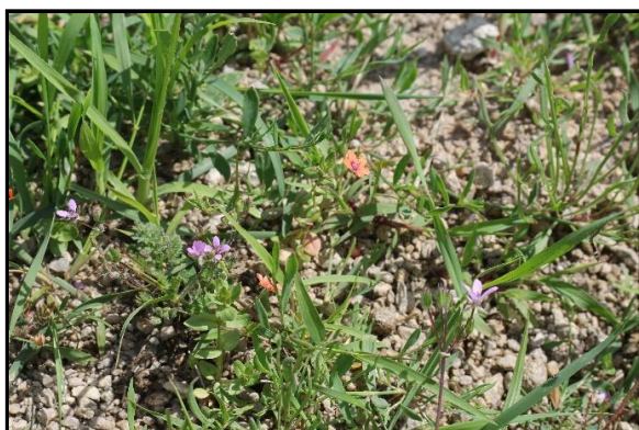
Obr 15 a 16: Červnová vegetace jednoletého úhoru suchých stanovišť – vlevo Fládnitzská chata s druhy pumpava rozpuková ( Erodium cicutarium ) a bér zelený ( Setaria viridis ), vpravo Zimmerhakelova step – porost merlíku bílého ( Chenopodium album ).
