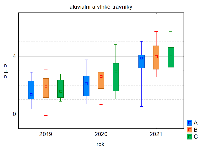
Obr. 33, 34 a 35: Hodnoty PHP vypočítané pro jednotlivé typy porostů.
