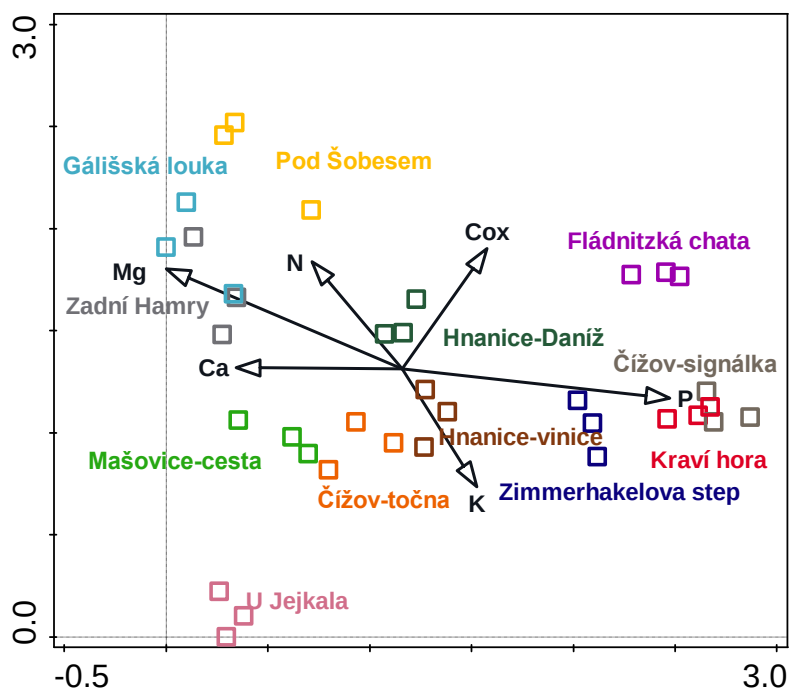
Obr. 6: Ordinační diagram DCCA zobrazující odběrové plochy (čtverce) na jednotlivých lokalitách (znázorněno různými barvami) ve vztahu k chemismu půd (černé vektory). Diagram znázorňuje rozdělení lokalit do skupin dle vlhkosti, pH a živin v půdě (hlavní gradient na první ose, vlhčí louky vlevo, z toho aluviální vlevo nahoře, ostatní vlevo dole a uprostřed, suché acidofilní trávníky vpravo), jak jsou prezentovány v dalších výsledcích.
